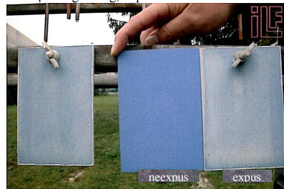
Vopsea acrilică pentru fațadă, locație Magdeburg, după 4 ani
