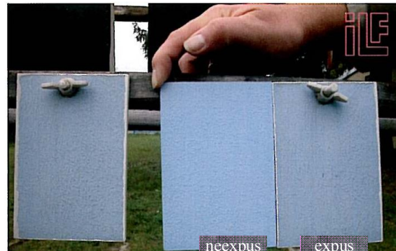
Vopsea pentru fațadă pe bază de silicon cu "efect lotus" Locație Magdeburg, după 4 ani
