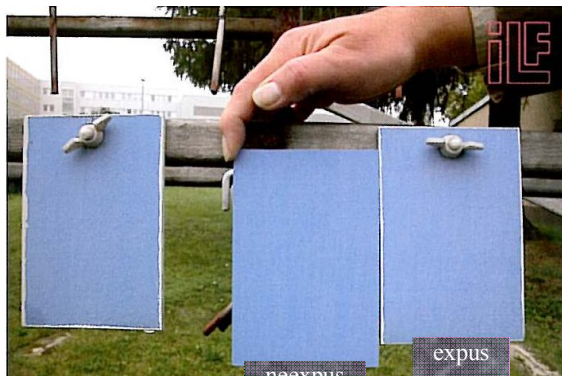
KEIM Granital, locație Magdeburg, după 4 ani
