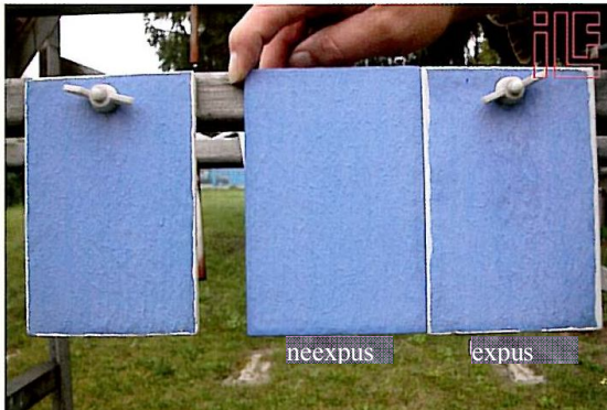
KEIM Purkristal, locație Magdeburg, după 4 ani
